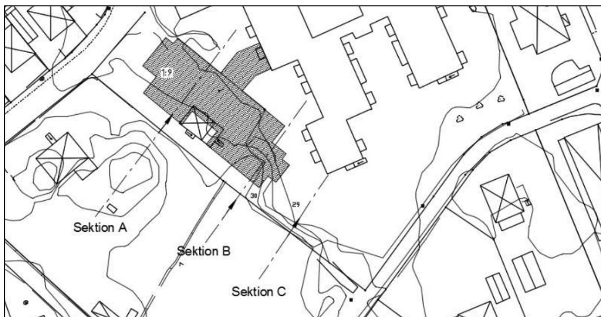
Figur 10-8 – Beräknade stabilitetssektioner benämnda Sektion A–C (ÅF, 2017).
